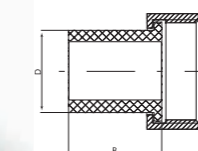
Штуцер с накладной гайкой
