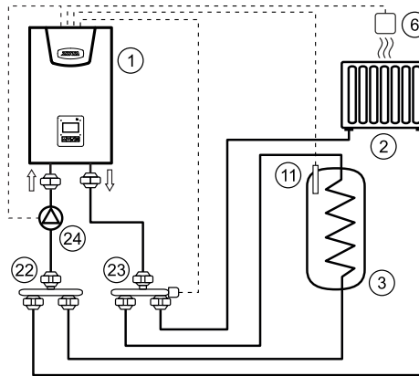
Рис.10 Упрощённая схема подключения котла в режиме «Отопление-ГВС».
