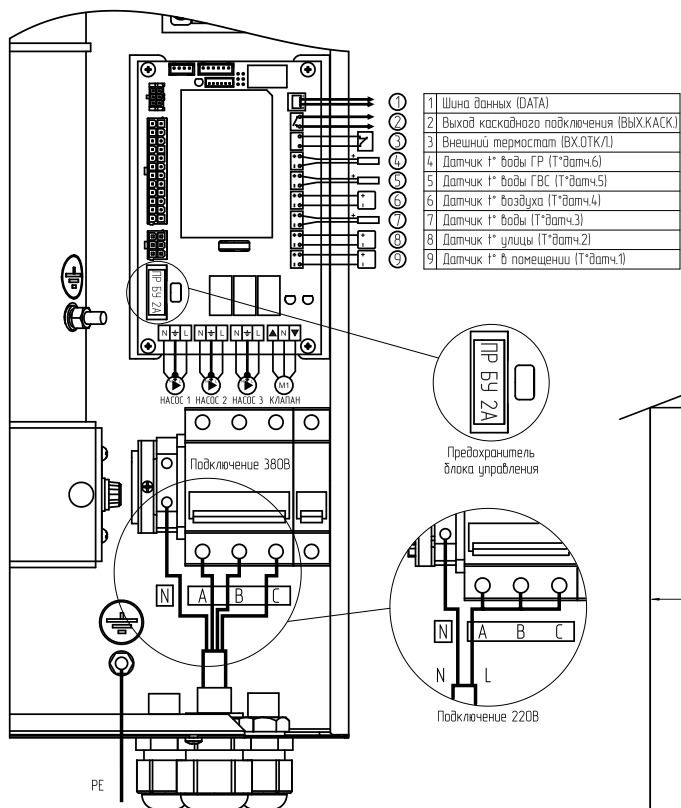
Рис.3 Схема подключения котла
