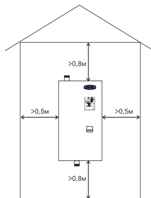
Рис.4 Схема установки котла
