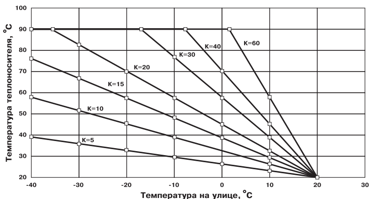
Рис.9 График погодозависимого регулирования
