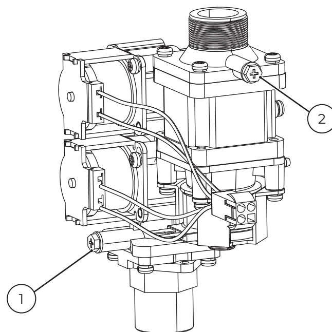
Рис. 40. Газовый клапан.
