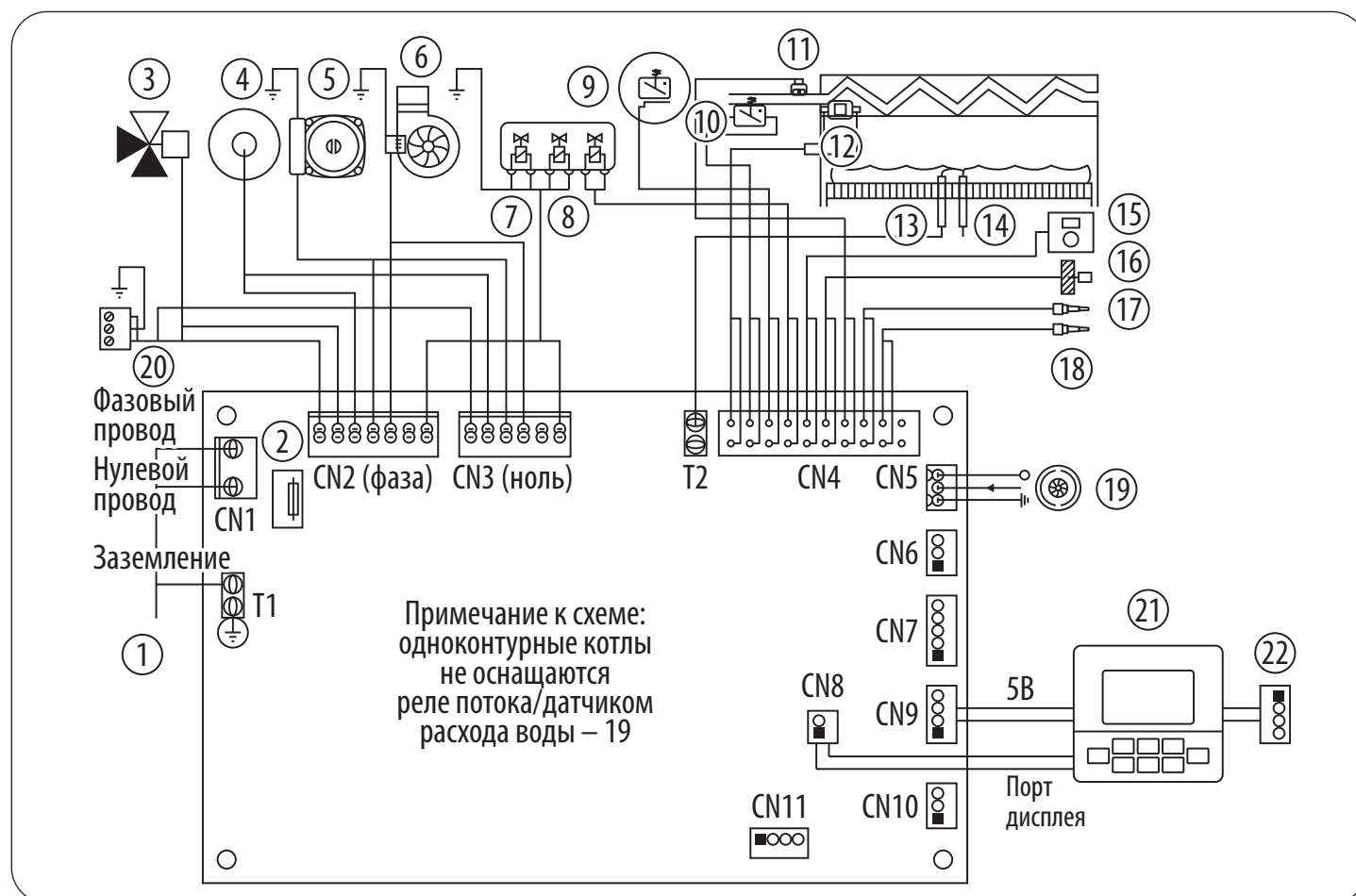
Рис. 46. Электрическая схема.
