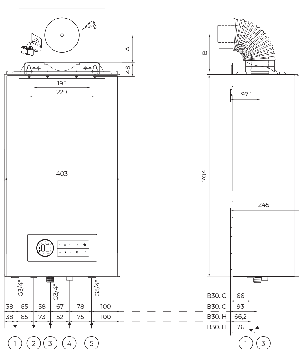
Рис. 42. Монтажные размеры B30 18 C/H, B30 24 C/H.
