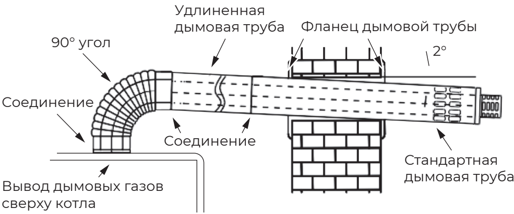
Рис. 45. Пример монтажа схемы C12.
