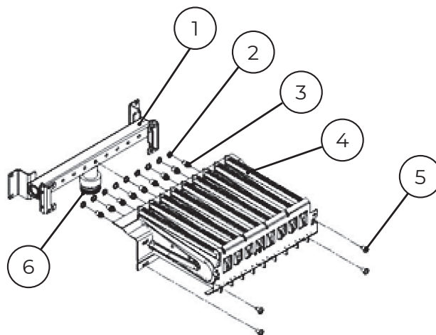
Рис. 39. Газовая горелка.
