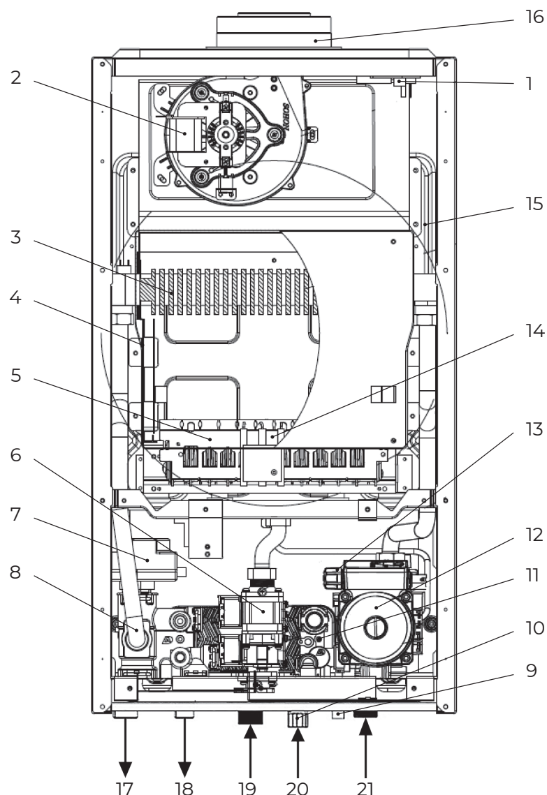
Рис. 3. Общая схема котлов B30 28 C, 32 C, 36 C.
