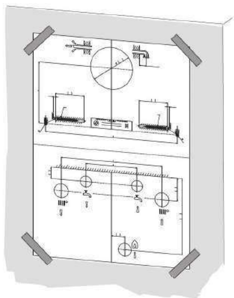
Рис. 31 Монтажный шаблон
